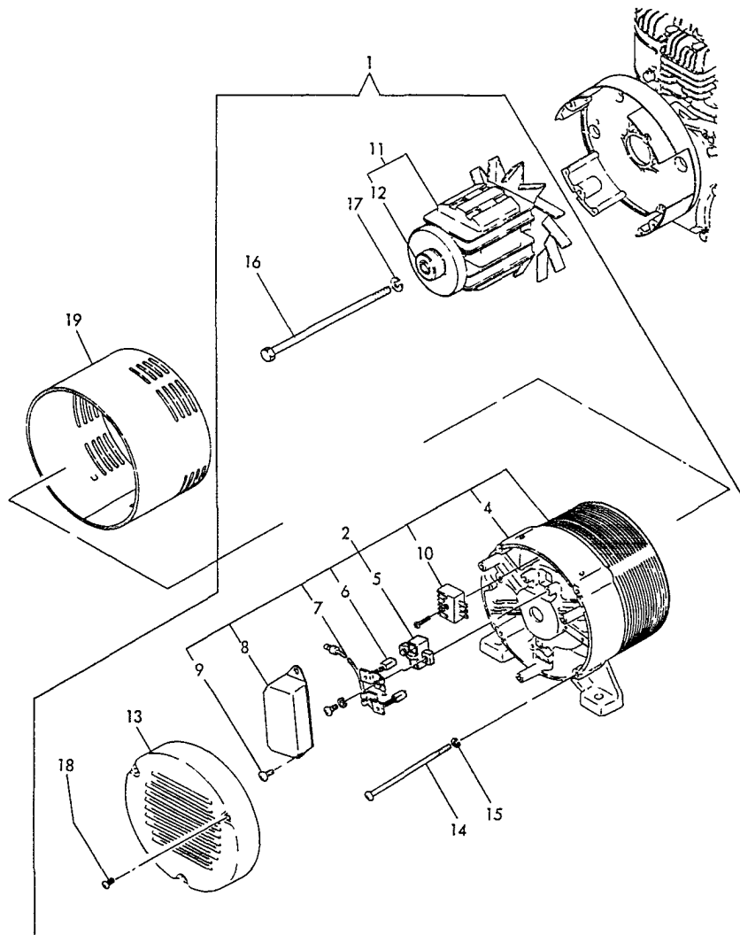
(16) GENERATOR
