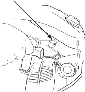
Tornillo de ajuste del ralentí
